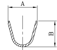
SEC A-A'
